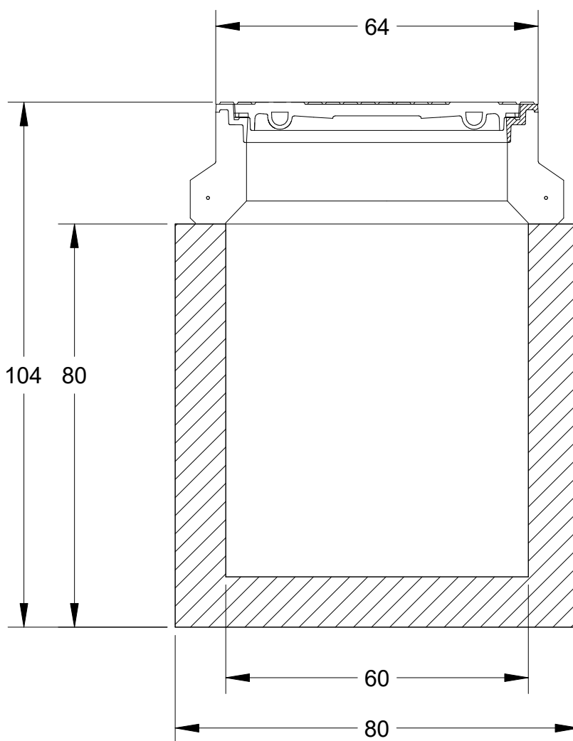
Betonput 80x80cm
